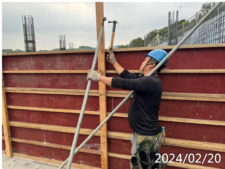
女寮2區1F柱牆模板組立
