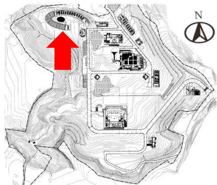
女寮1區噴漿護坡
