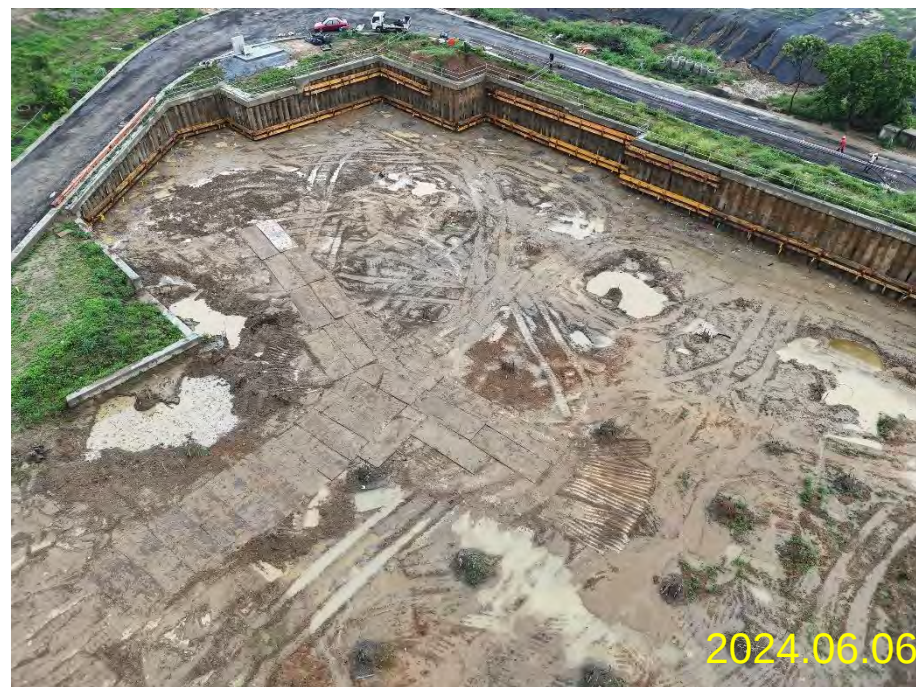
齋堂第二層地錨(圍令背填施作、施預力) 第三層土方開挖
