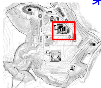
齋堂第二層地錨(圍令背填施作、施預力) 第三層土方開挖
