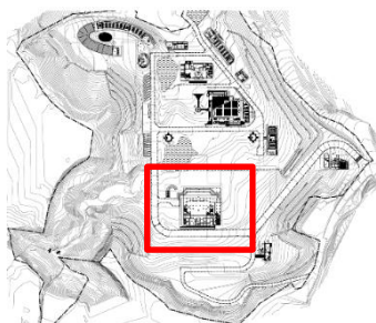
主殿PC打底、地梁放樣
